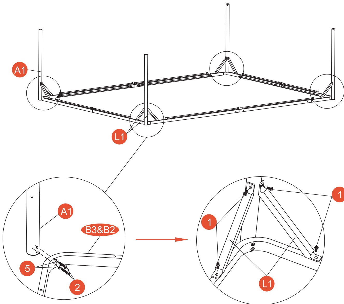
5 (8PCS) Ø17*Ø9.5*1.5
