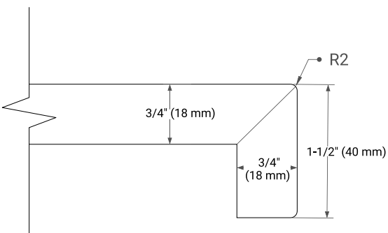
EDGE SIDE VIEW
