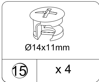
Cam lock Tornillo de cerradura Serrure de came TSF0305
