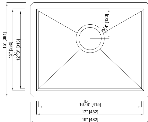
TOP
