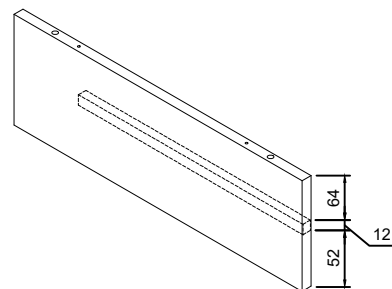
Left drawer divider Séparateur de tiroir gauche QTY: 1
