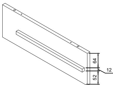
Right drawer divider Séparateur de tiroir droit QTY: 1
