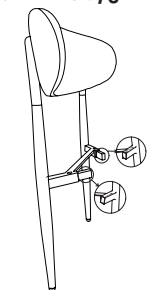
Rear Frame *1 Hinterer Rahmen *1 Telaio posteriore *1 Cadre arrière *1 Marco trasero *1 後部フレーム *1
