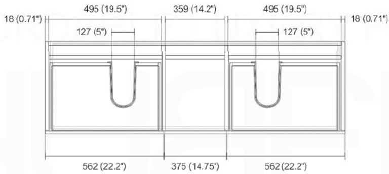
. TOP ELEVATION
