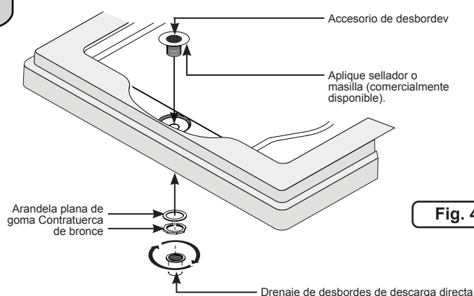
Figura 4: Instalación del sistema contra desbordes
