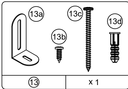
13 x 1 #A84050 safety bracket kit juego del soporte de seguridad ensemble de courroie sécurite
