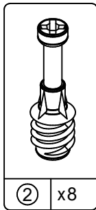
② x8 #A22610 cam bolt perno de leva boulon de came
