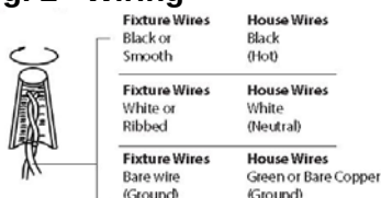
Fig. 2 Wiring
