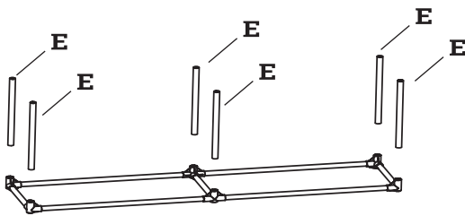
Assemble E
