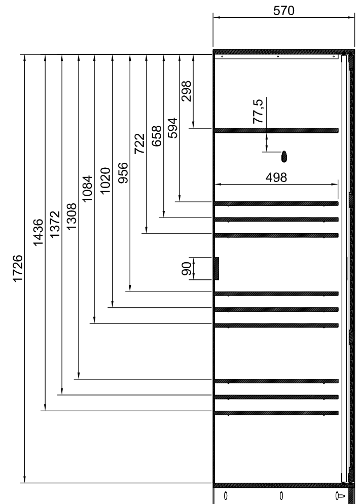
Corte A-A
