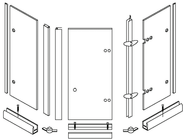
LEFT DOOR INSTALLATION
