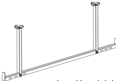
Assemblage de la barre de suspension MAX 50 lb/Assemblage
