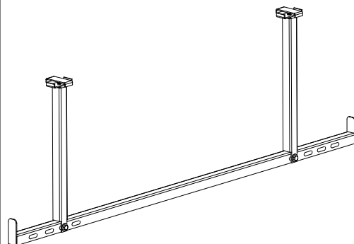
Assemblage de la barre de suspension
