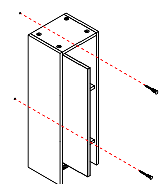
Left door opening
