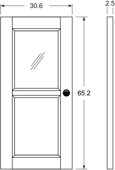
DOOR DETAIL
