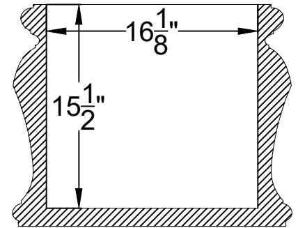
SECTION A-A1
