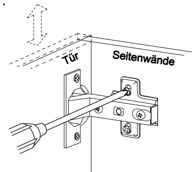
Vertical Über die Schlitzlöcher in der Halterungsplatte oder über Nockenverstellung
