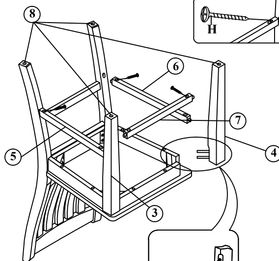
DÉTAIL D
