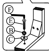
DÉTAIL A
