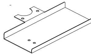
Placa de montaje para el receptor
