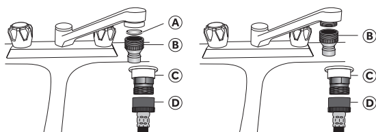
Filetages Internes
