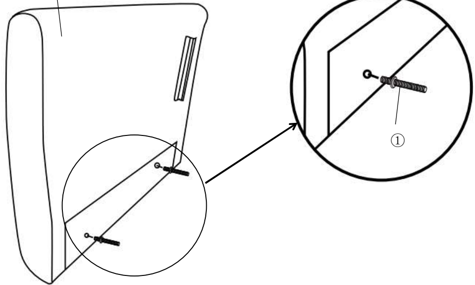
Left Armrest(B)
