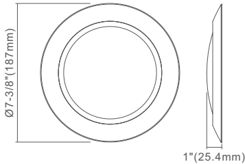
HB-DL6R15W3KWHIET
