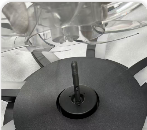
22 Install the fan blades.
