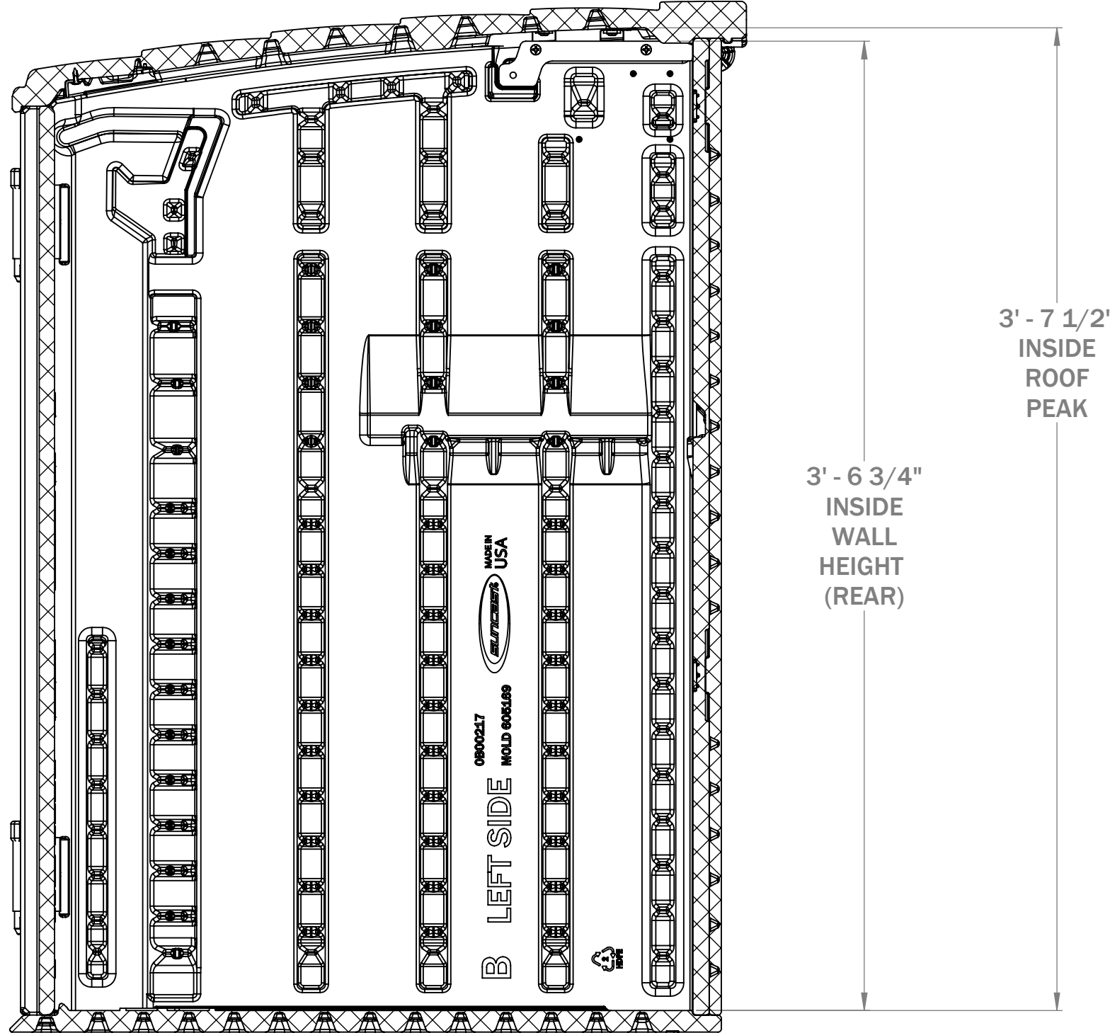
SECTION A-A SCALE 1 : 6
