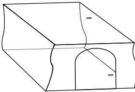
B-300X300X245mm(1pc)
