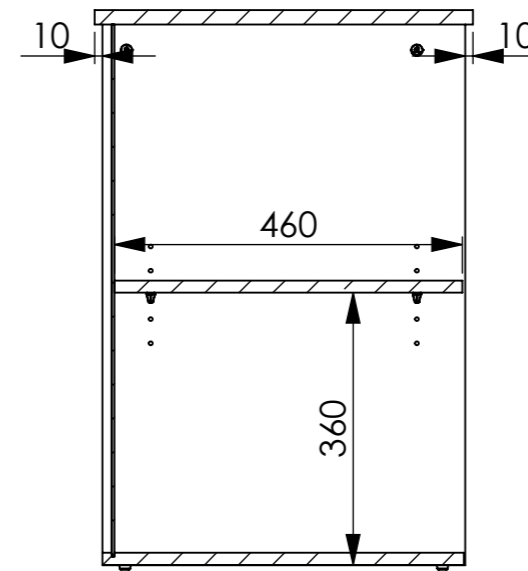
COUPE A-A
