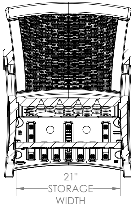
SECTION B-B SCALE 1 : 12
