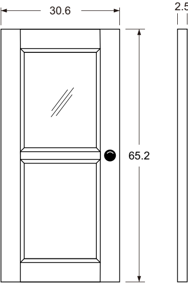
DOOR DETAIL
