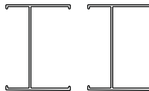
Wall Jamb(2)
