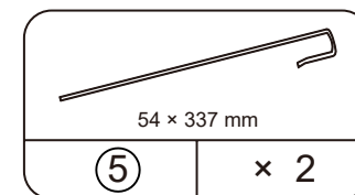
HOOK
