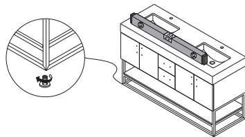
2. Adjusting cabinet foot/Pieds de cabinet de réglage
