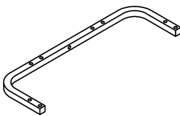
Top U-Frame
