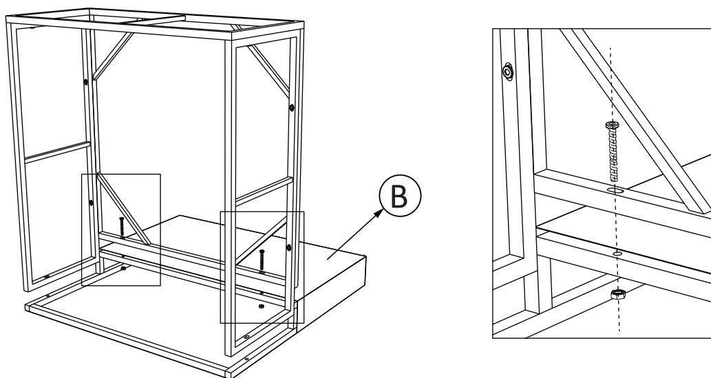
Bolt M6x50
