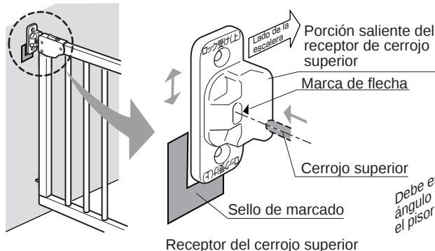
Receptor del cerrojo superior
