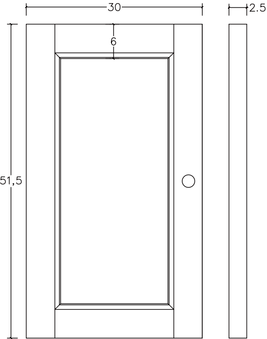
DETAIL DOOR
