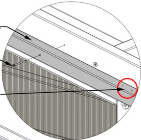
P02 (x2) PURLIN CLEAT
