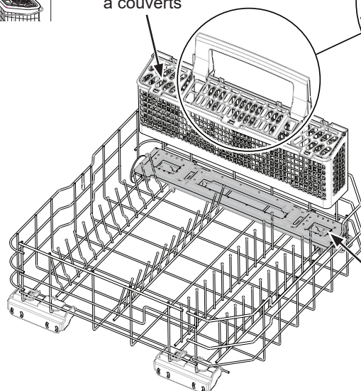
Couvercles des paniers à couverts
