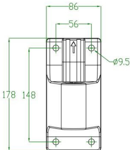
Orificio para soporte de pared de plástico
