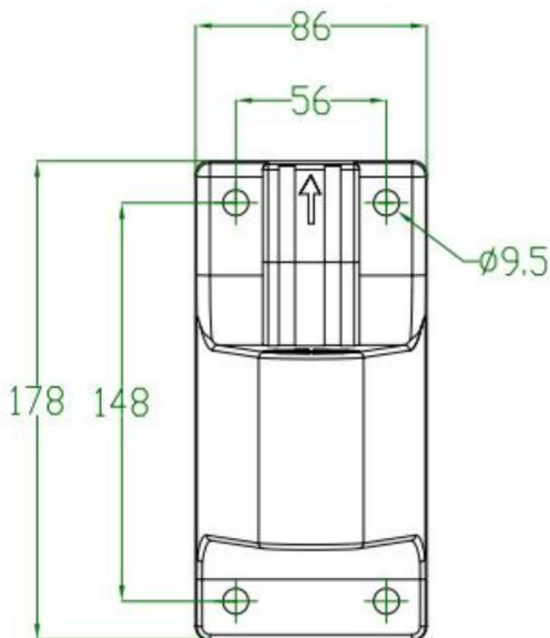
Loch für Kunststoff-Wandhalterung
