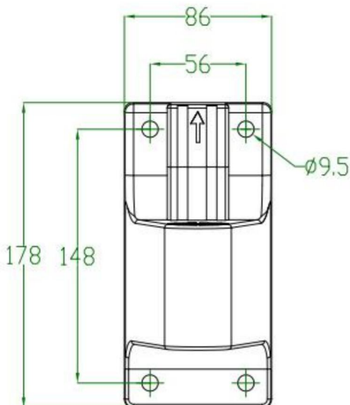
Otwór na plastikowy uchwyt ścienny
