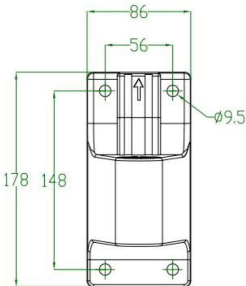
Gat voor kunststof wandbeugel
