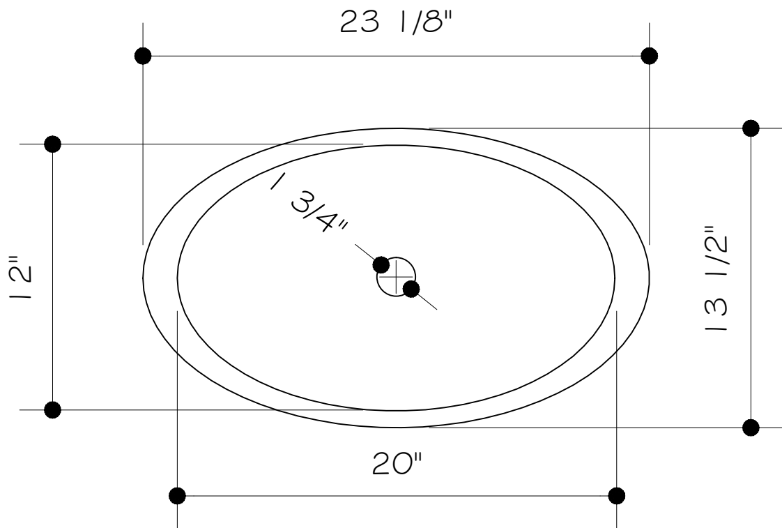
VISTA SUPERIOR
