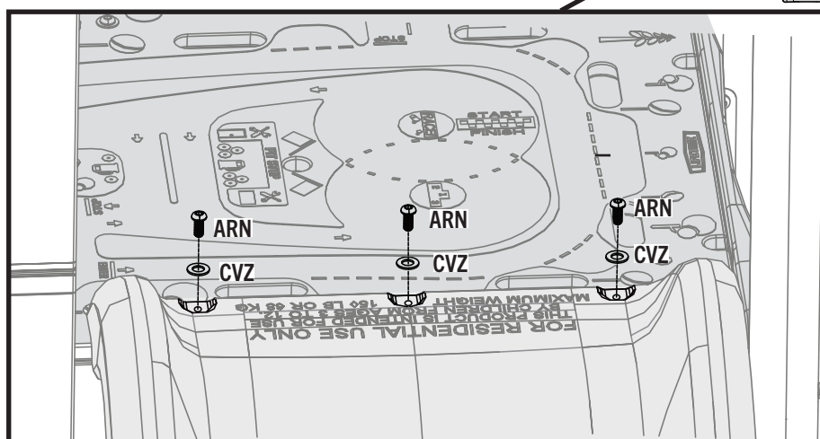
Top of deck view / Vue du dessus des ponts / Vista superior de la plataforma
