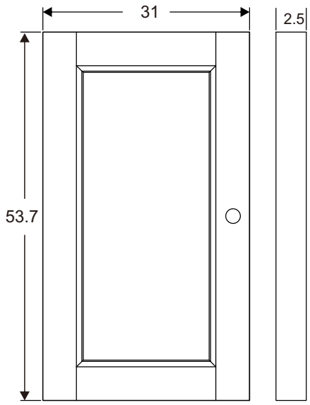
DOOR DETAIL
