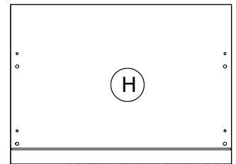
CS3106 397x548x22mm
