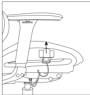
Griff anheben zur Einstellung der Sitzhöhe.
