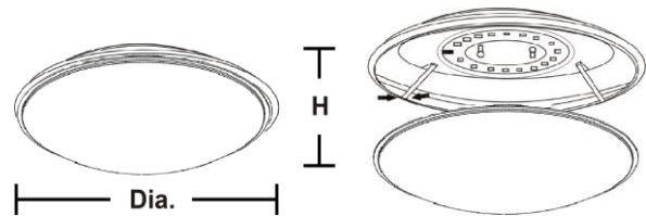
Dia.=13" / 17" H=3.5"
