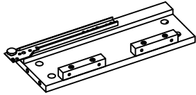
Side frame table (right) - 1pc Table à cadre latéral (droite)
