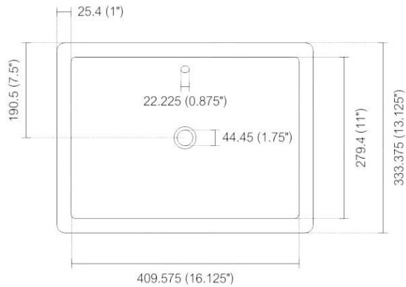
TOP ELEVATION
