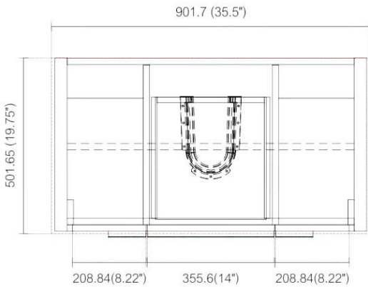
TOP ELEVATION
