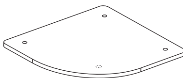
E 390*390*12mm(2pcs)
