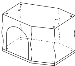
B 400*300*12mm(1pc)
