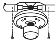
FIGURE - 4 MONTAGE PAR LA TIGE INFÉRIEURE SEULEMENT
