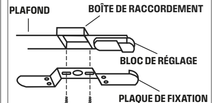
FIGURE - 5 MONTAGE ENCASTRÉ SEULEMENT
