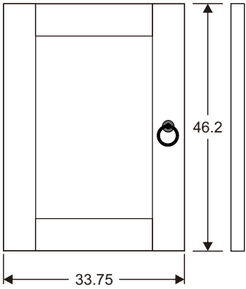
DOOR DETAIL
